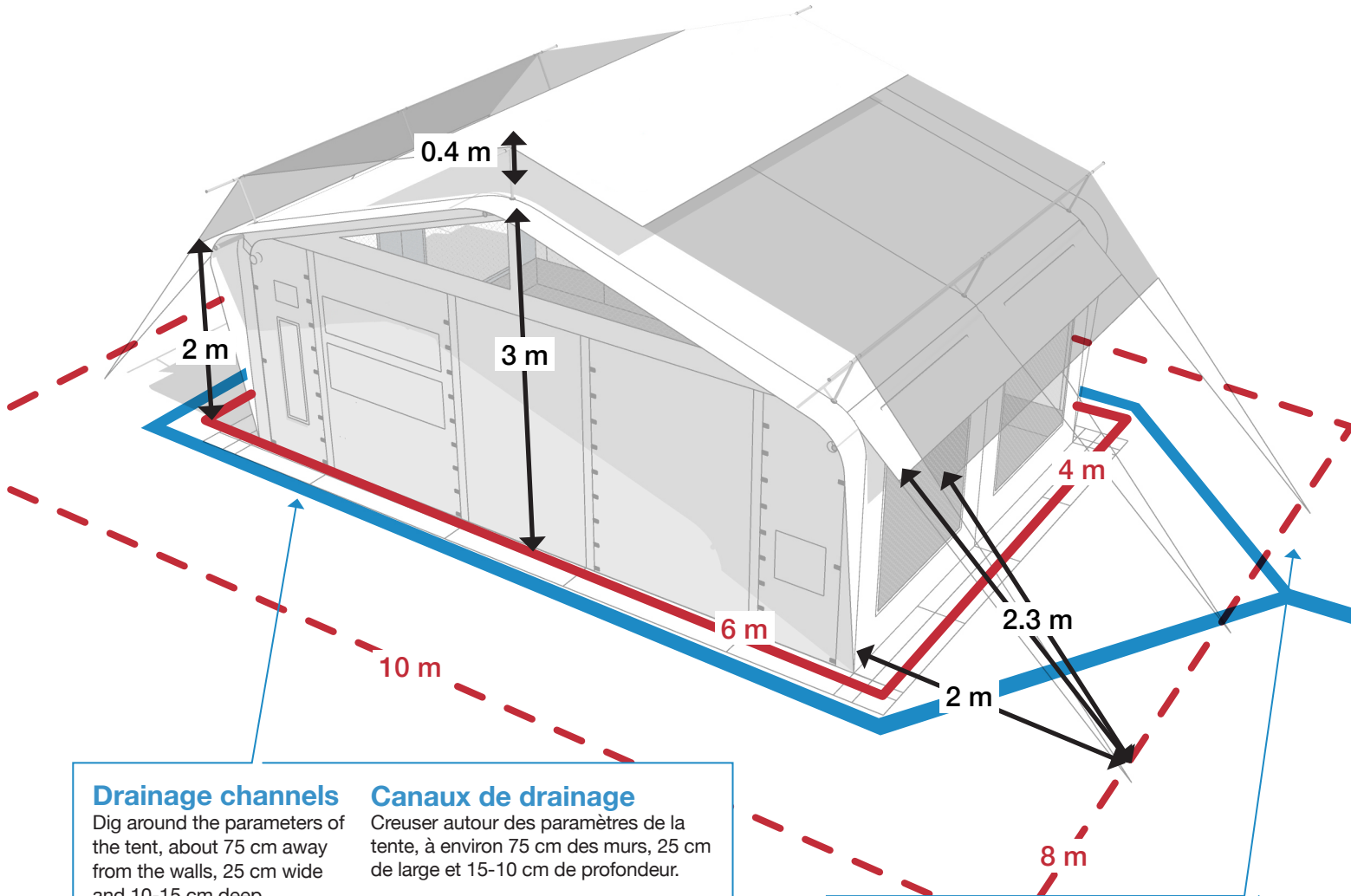
Site dimension Dimension du site Dimensiones del emplazamiento قياس الموقع
